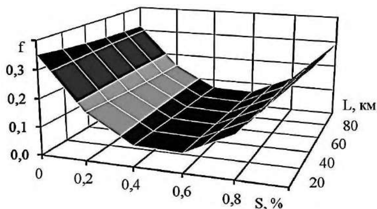
Рис. 2. Изменение коэффициента трения f от концентрации серы S и пути трения деталей L
