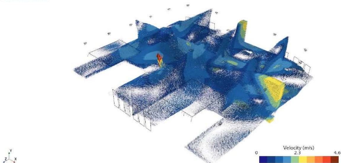
Рис. 13. Векторное отображение скоростей потоков газов в горизонтальном сечении помещения.
