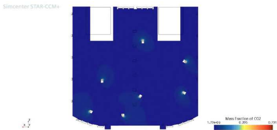
Рис. 7. Массовая доля CO 2 в горизонтальном сечении помещения.
