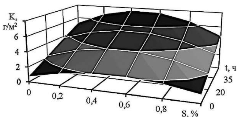
Рис. 1. Изменение коррозионности моторного масла K от содержания серы S и продолжительности испытания t
