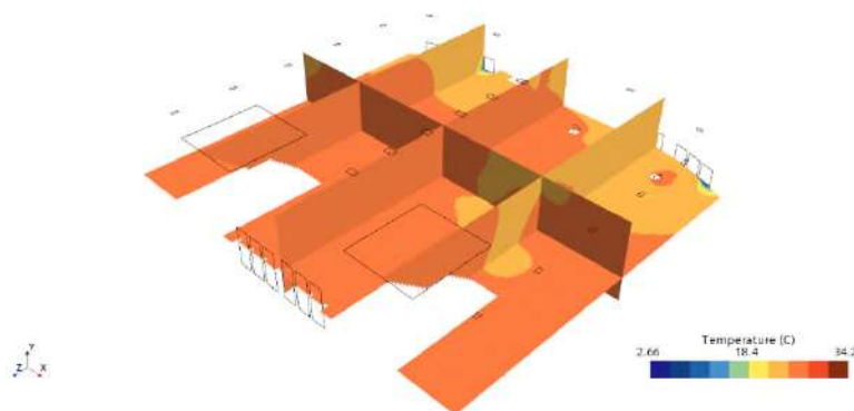
Рис. 10. Распределение температур в изометрии.
