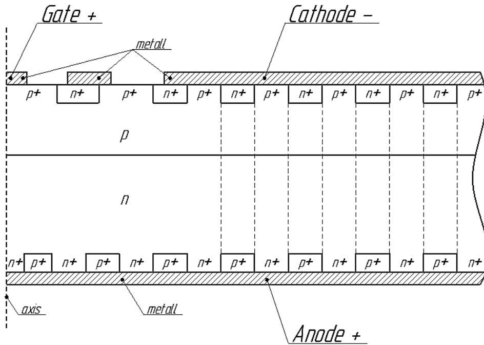
Рис.3 Динистор с интегрированным шунтированным управлением прямой полярности.
