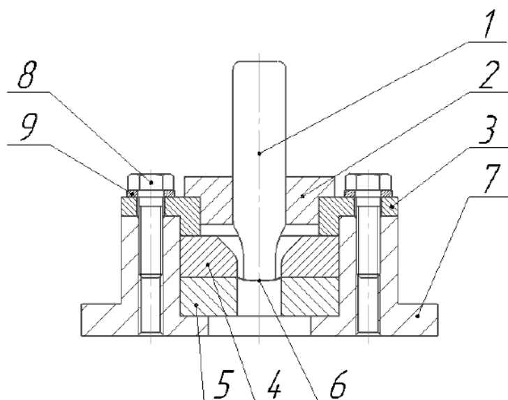
Рис. 2. Эскиз лабораторного штампа для формовки контакта: 1 – пуансон; 2 – направляющая втулка; 3 – прижим; 4 – кольцо; 5 – матрица; 6 – заготовка; 7 – основание; 8 – болты; 9 – шайбы
