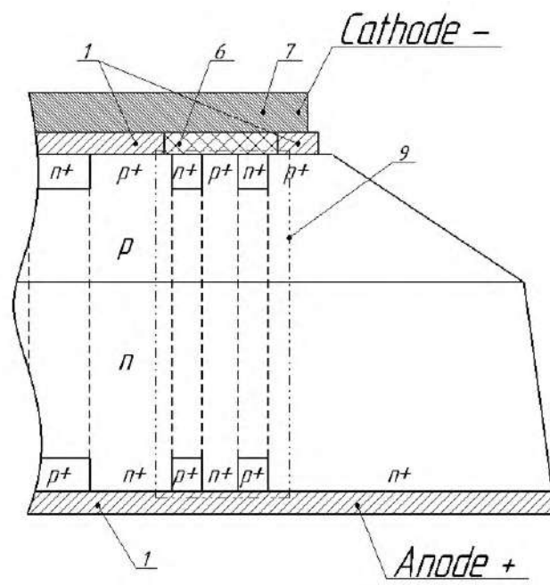
Рис.6.2 Краевая область динистора прямой полярности с разделением металлизации 9 кольцом n^+-n-p^+- структуры между двух колец p^+-n-p^+- структур.
