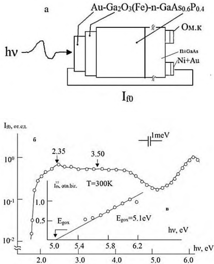
Рисунок 1. Схема исследуемой наноструктуры Au-Ga 2 O 3 (Fe)-n-GaAs 0.6 P 0.4 (а) и ее спектральные характеристики (б), определение фотоэлектрическим методом ширины запрещенной зоны ( E_{gox} ) оксидного слоя Ga 2 O 3 (Fe), сформированного на GaAs 0.6 P 0.4 -полупроводнике (в).
