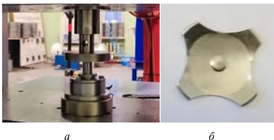
Рис. 3. Деформация заготовки в штампе (а) и внешний вид образца (б)
