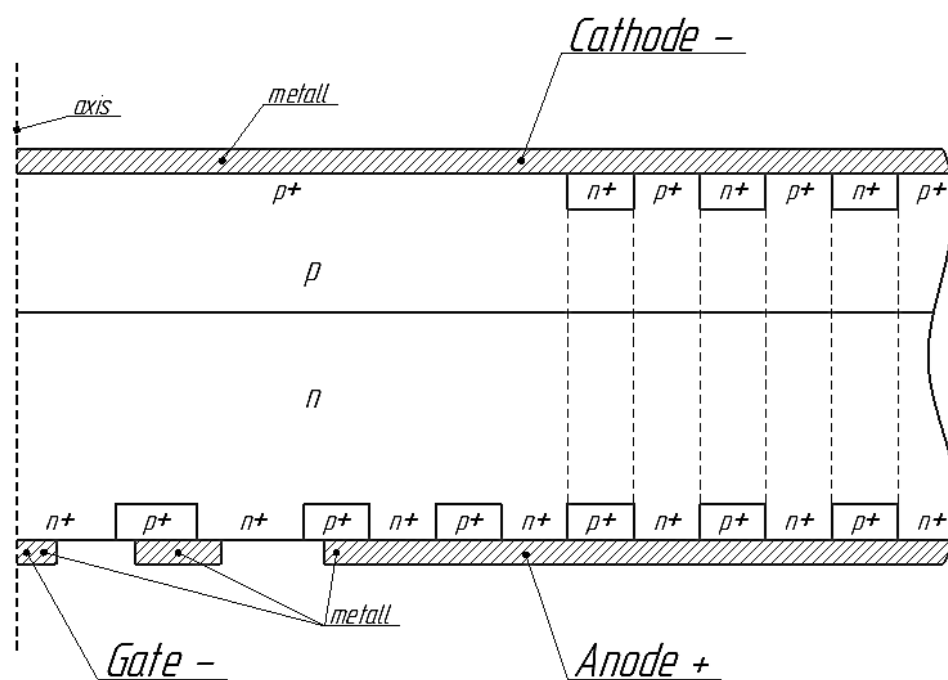
Рис.1 Динистор с интегрированным управлением прямой полярности.
