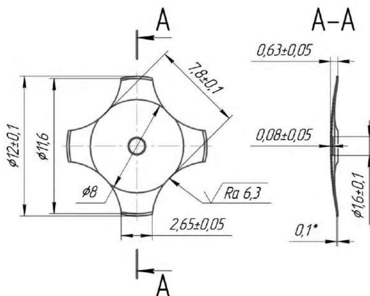
Рис. 1. Эскиз детали «Контакт»
