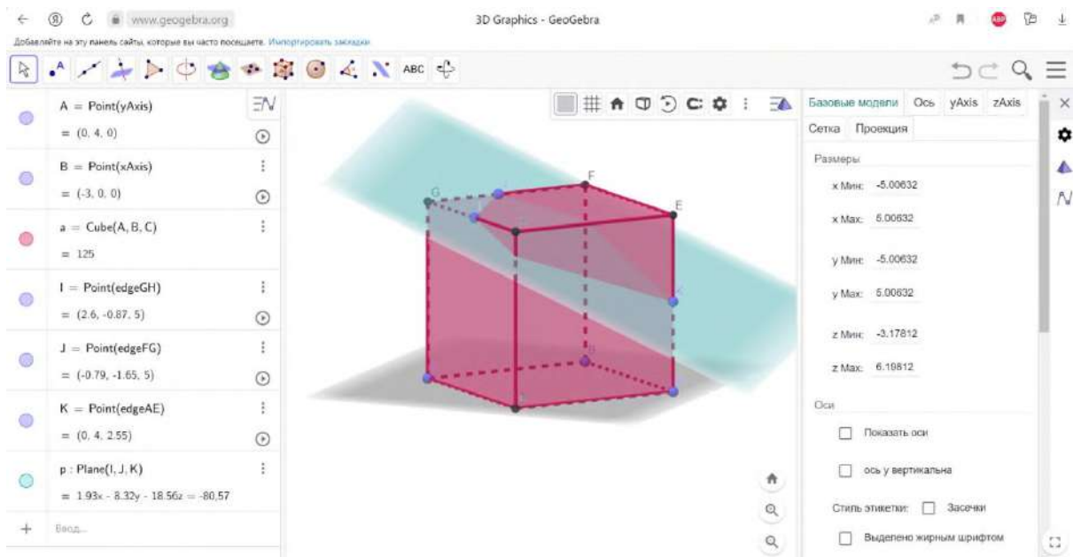
Рис. 1 Пример построения сечения куба по трём точкам.
