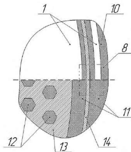
Рис.7 Динистор прямой полярности с разделением металлизации кольцом p^+-n-p^+- структуры 8, вид краевой области со стороны катода:
