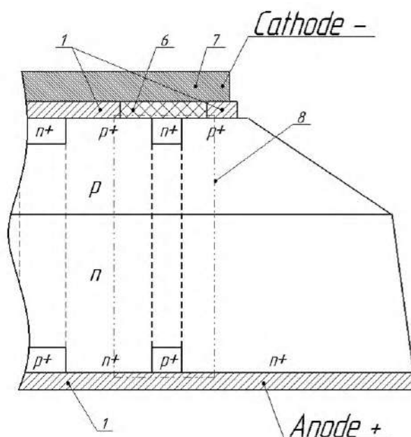
Рис.6.1 Краевая область динистора прямой полярности с разделением металлизации 8 кольцом р+-n-p-n+-структуры.
