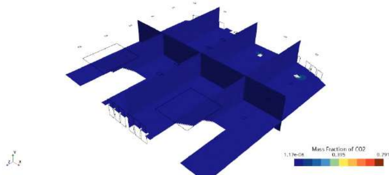
Рис. 12. Массовая доля CO2 в объеме.
