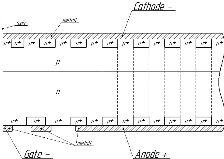
Рис.4 Динистор с интегрированным шунтированным управлением обратной полярности.
