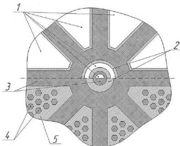
Рис.5 Динистор с интегрированным управлением прямой полярности, вид со стороны катода: вид сверху – структура с металлизацией 1, вид снизу – структура без металлизации 1.
